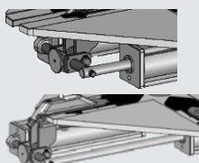
Sistema FLEX de cierre con mordazas ajustables (capacidad 10" ÷ 27")
